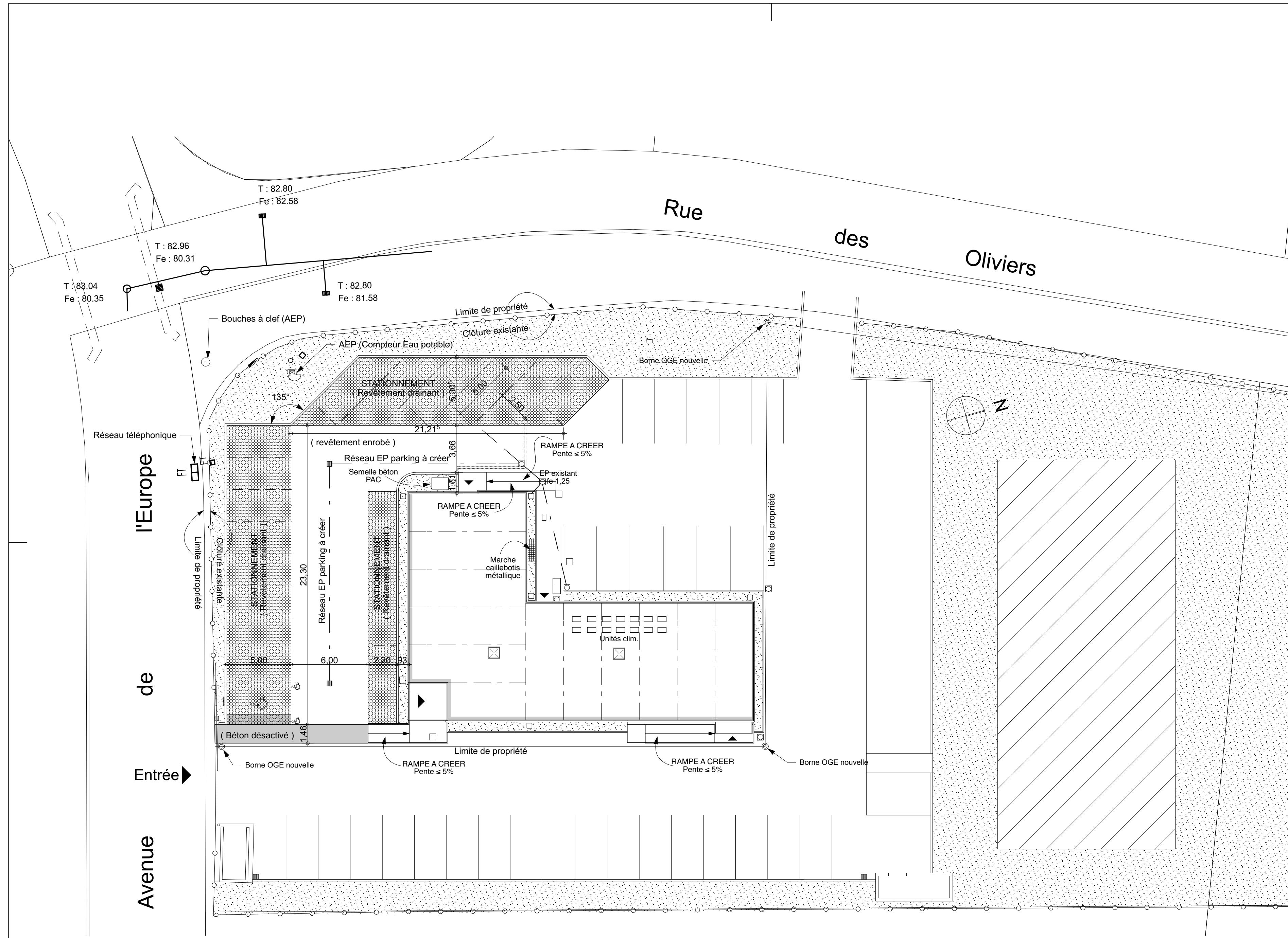
PLAN MASSE PROJET - ECH 1/200
